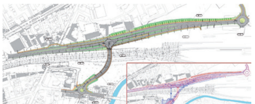
Planimetria del cavalcaferrovia di Via Maganza.
